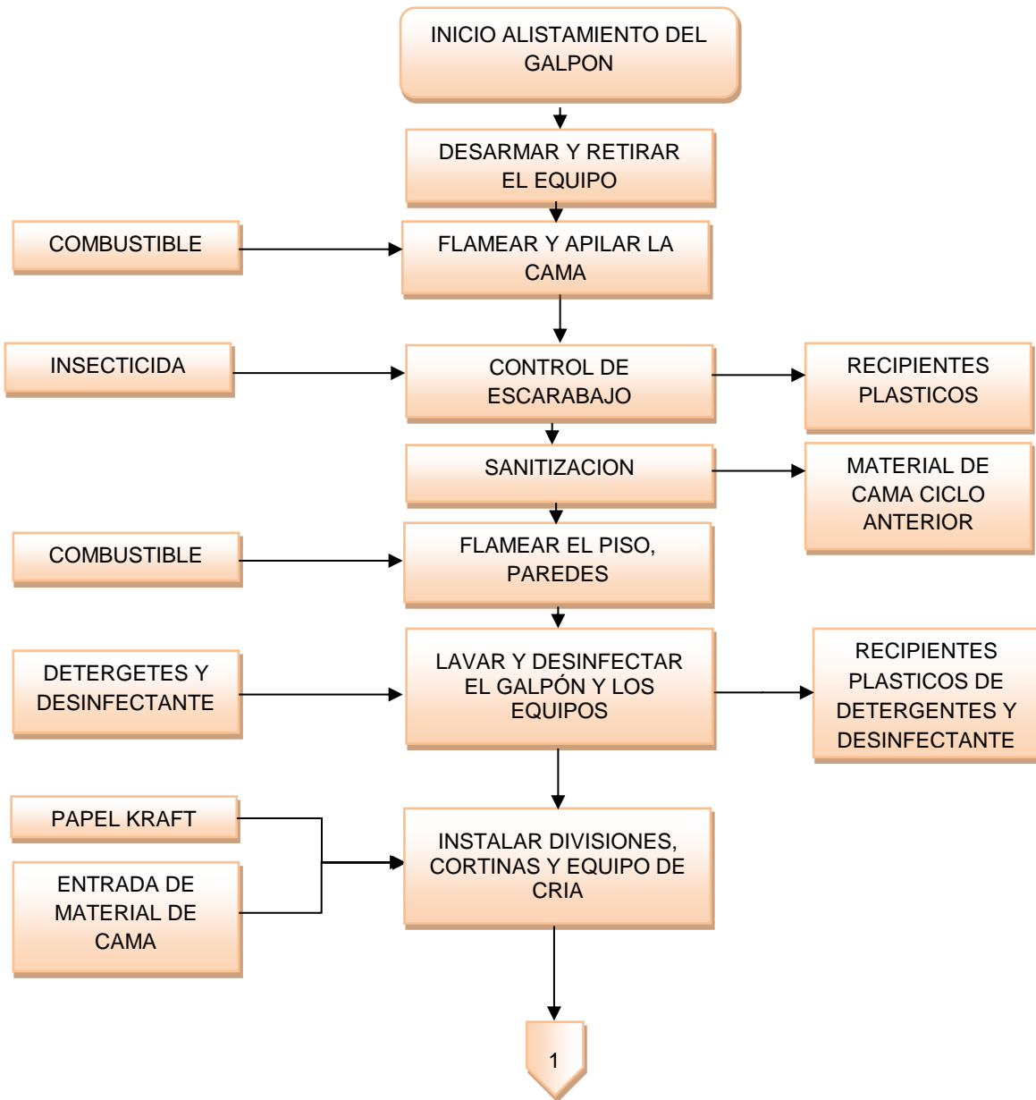
Figura 1. Diagrama de Flujo Granja Avícola El Placer
